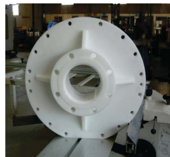
TORNILLOS DE ARRASTRE / TAPAS
